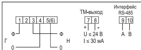
Рисунок В.13 – Схема включения счетчиков CE 102 тип корпуса R5, исполнения «АК»
