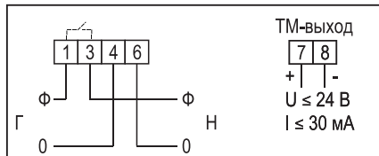
Рисунок В.5 – Схема включения счетчиков СЕ 102 тип корпуса S7, исполнения ОКРQVZ», «JR1KVZ», «JPKVZ», «JKR1QVZ», «JPKQVZ», «JKR1PQVZ»
