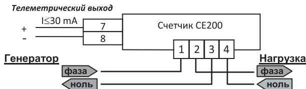
Маркировка схемы включения счетчика CE 200
