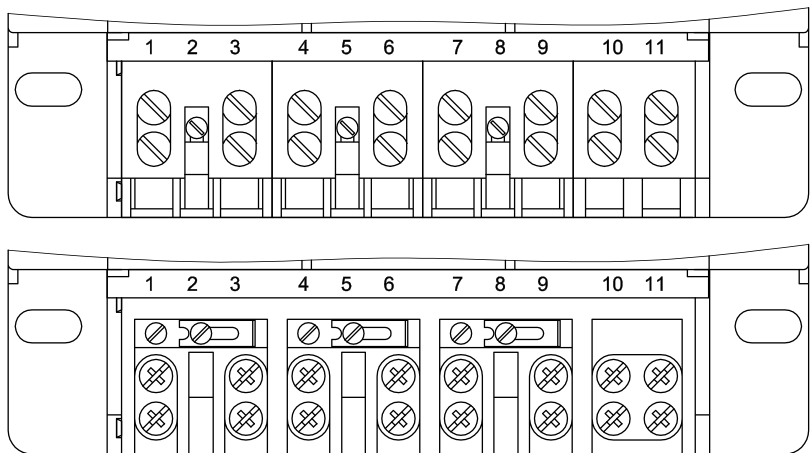
д) – обозначение контактов зажимов счетчика СЕ303 S31 74Х
