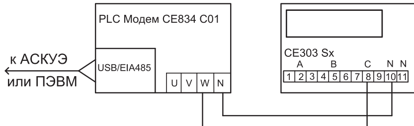
Рисунок 3.10 – Схема подключения счетчика
