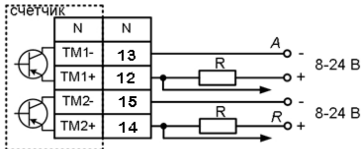
Рисунок Б.2 – Схема подключения электрических испытательных выходов счетчика
