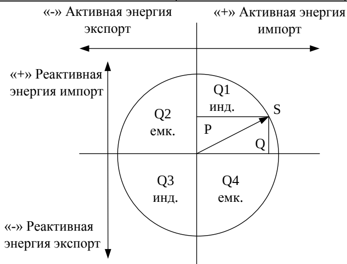
Рисунок 3.15 – Диаграмма распределения активной и реактивной энергий по квадрантам
