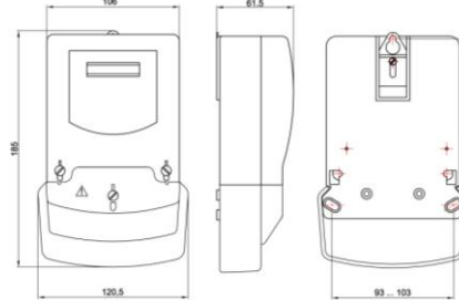
(тип корпуса Ш4)
