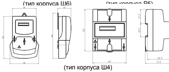
(тип корпуса Ш4)
