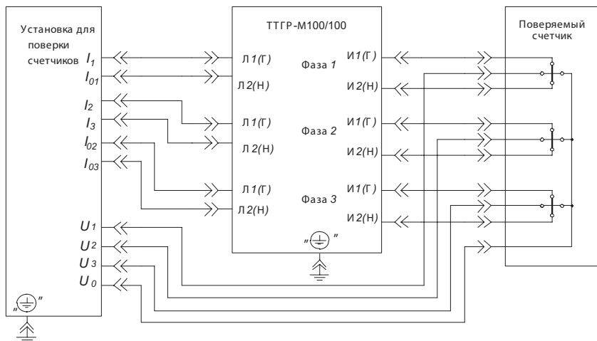
Рисунок 4.4 – Схема соединений при поверке трехфазного четырехпроводного счетчика с изолированными последовательными и параллельными цепями (каналы тока источника тока изолированы).
