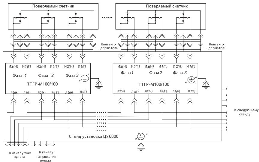
Рисунок 4.4 – Схема соединений при поверке трехфазного четырехпроводного счетчика с изолированными последовательными и параллельными цепями (каналы тока источника тока изолированы).
