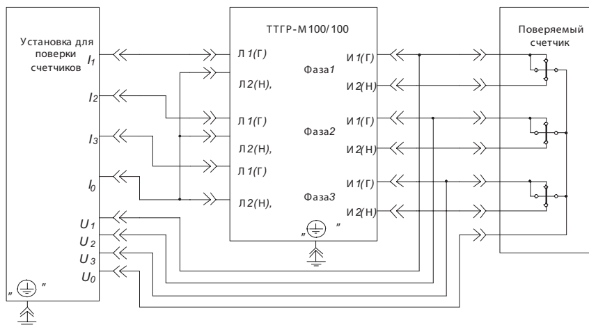
Рисунок 4.1 – Схема соединений при поверке трехфазного четырехпроводного счетчика с гальванически соединенными последовательными и параллельными цепями (каналы тока источника тока соединены «звездой»).
